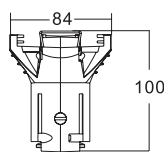
レンズ鏡筒 e19° X40268 e26° X40269 e36° X40274
